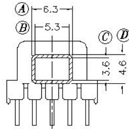
A-A SECTION
